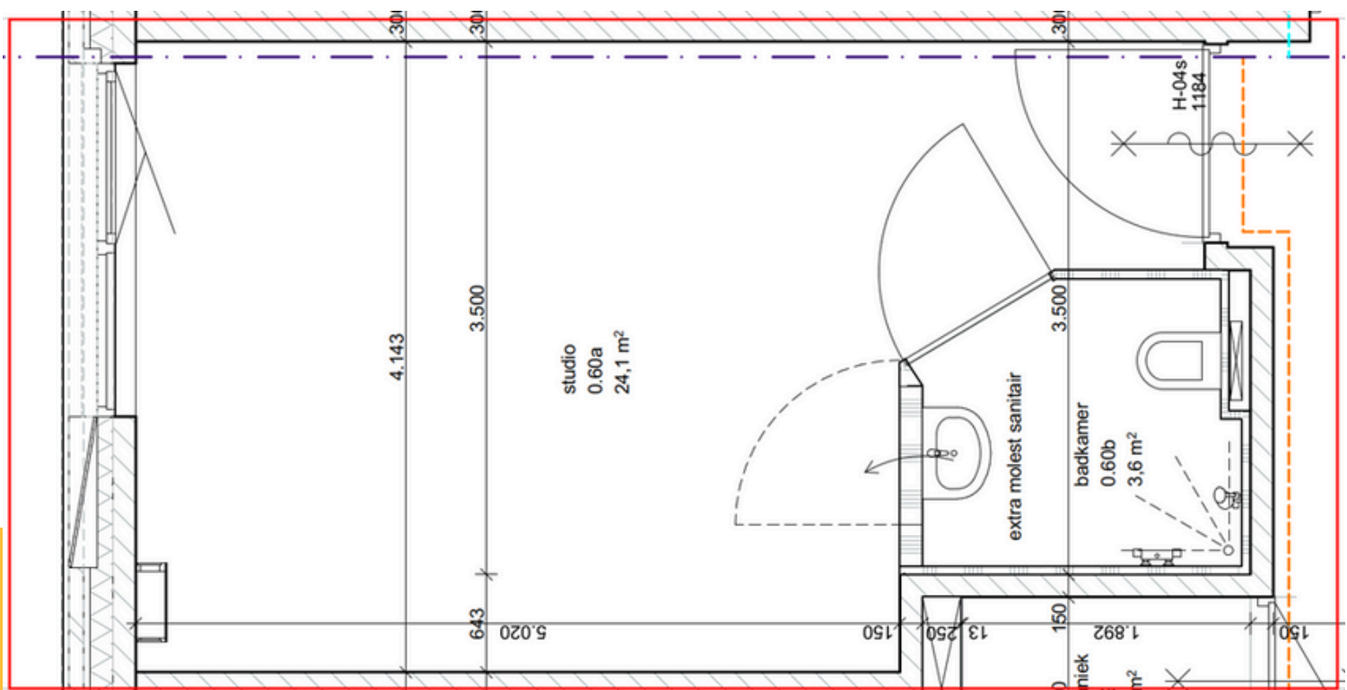
Afmetingen studio
