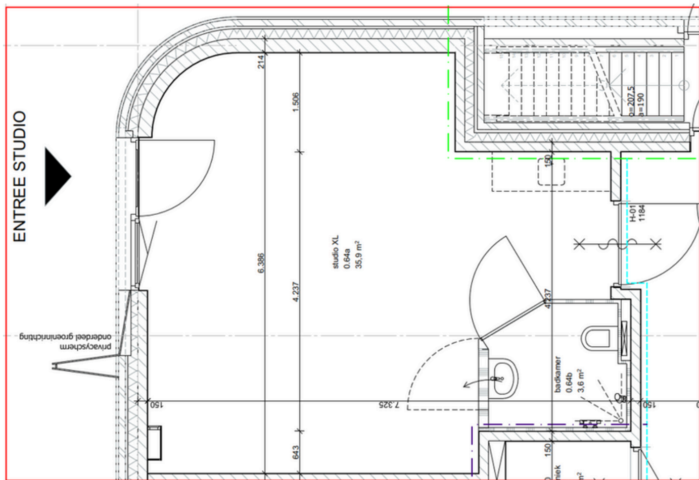
Afmetingen aanleunstudio
